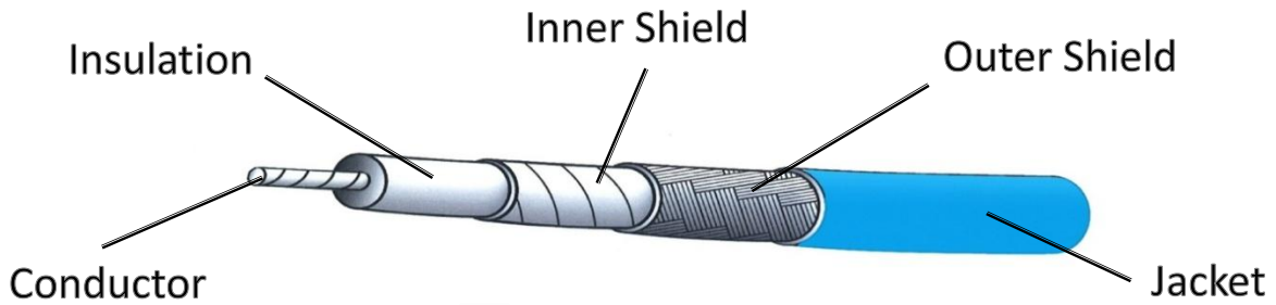
Actual Cable Section Illustration
